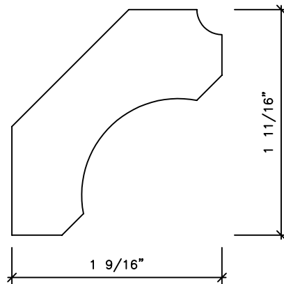
AC6016 7/8 x 2 1/4
