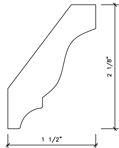
AC6017 5/8 x 2 5/8
