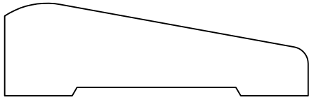
AC1001 11/16 X 2 1/4
